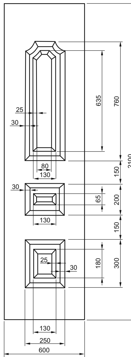
620 x 1680mm Minimální rozměry Min. size Min. Ausmass Dimension minimales
