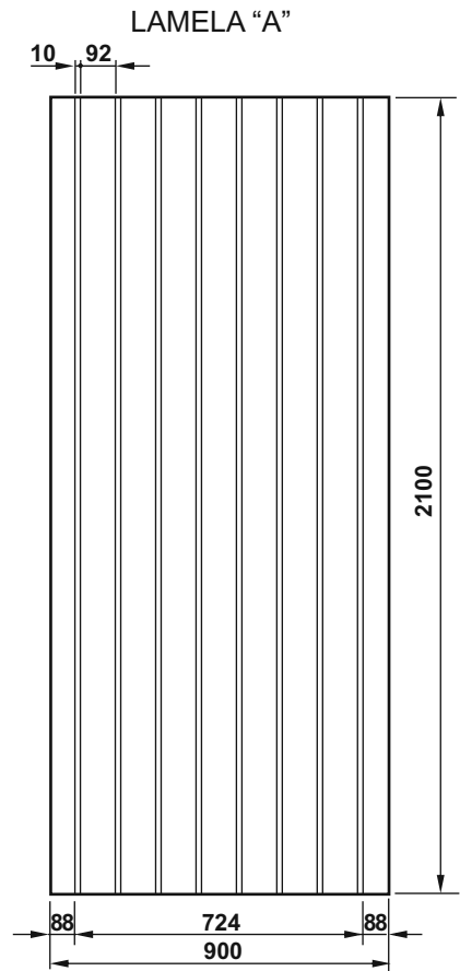
hloubka prolisu = 2 mm offset depth Tiefe der Versetzung (Einpresstiefe) profondeur l' moulage
